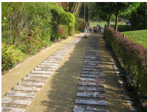
Accès carrossable en forte pente, dolomies stabilisées et passage de roues en pavés décoratifs: la solution pratique.
